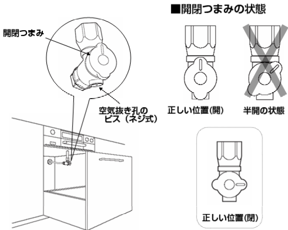
ガスコンロ用ガス栓の設置例
