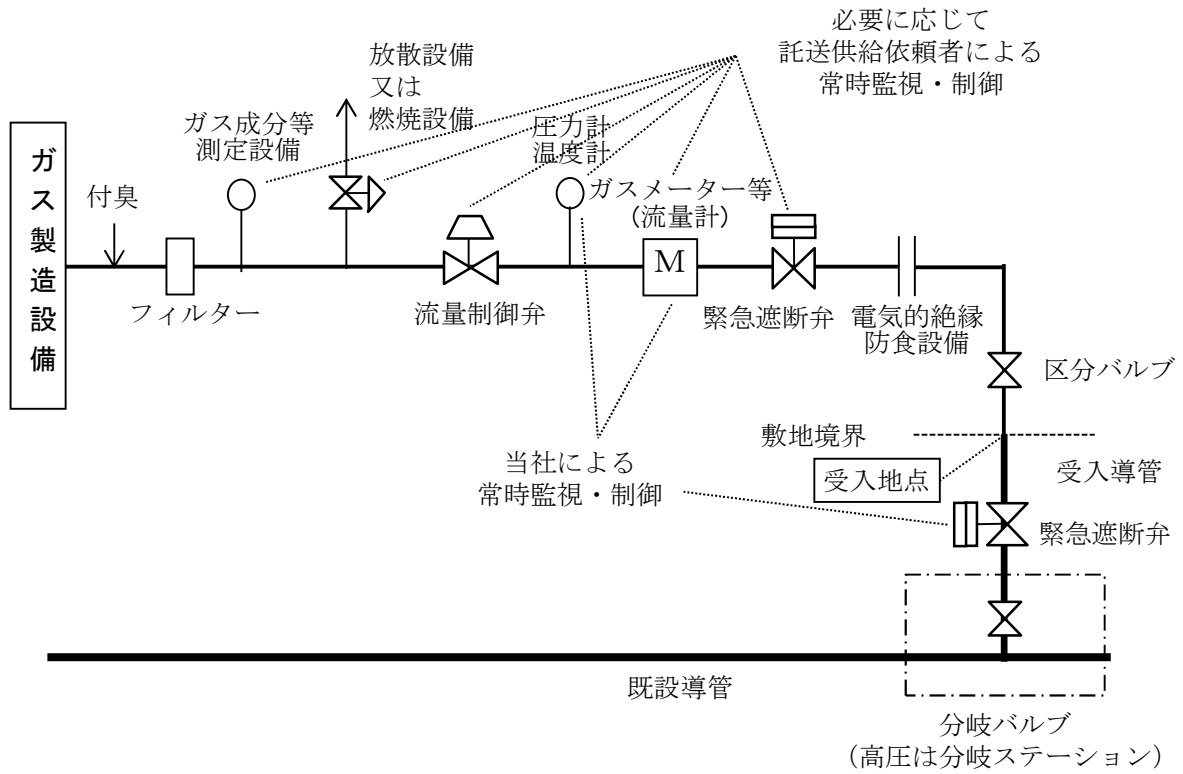
(参考) ガスの受入のために必要となる設備概要 (概念図)
